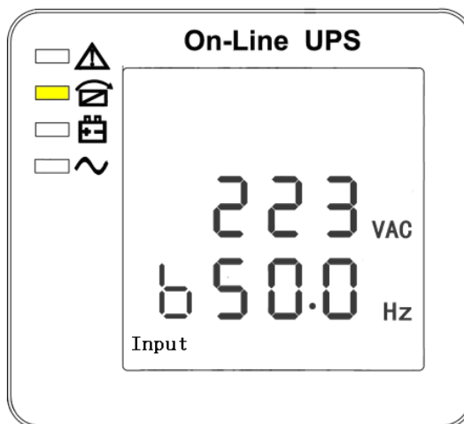
3. Фаза В (L2) Вход Напр. / Частота
