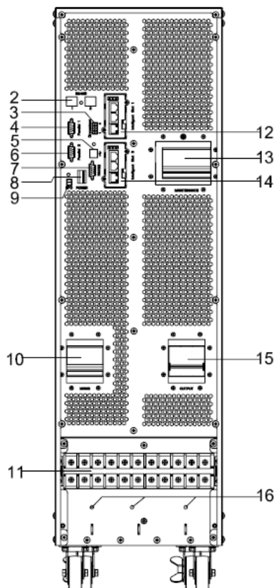
10-20 кВа вид сзади
