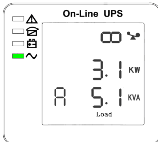
11. Фаза А (L1) Нагрузка
