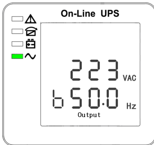
9. Фаза В (L2) Выход напр и частота
