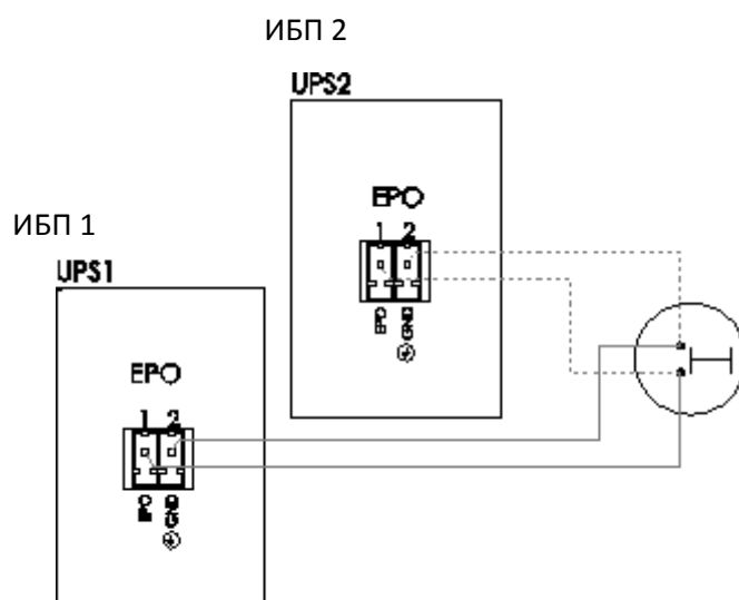
Схема подключения
