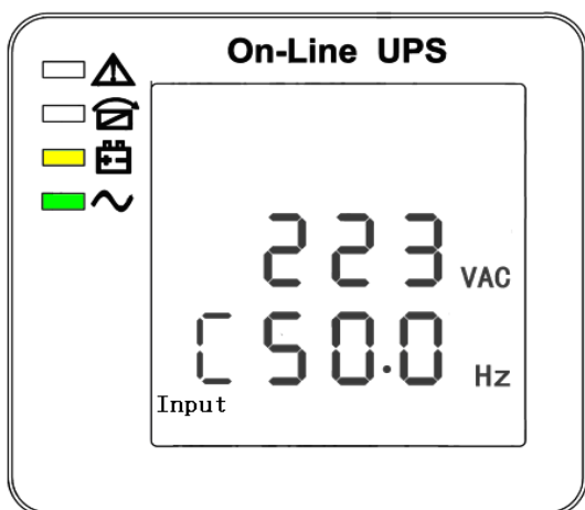
4. Фаза С (L3) Вход Напр. / Частота
